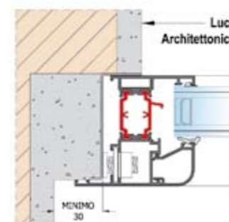
1. Sezione orizzontale - Nodo laterale fisso
