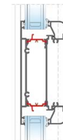
6. Sezione verticale - Nodo centrale
