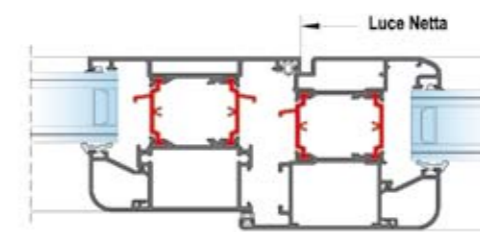
2. Sezione orizzontale - Nodo centrale
