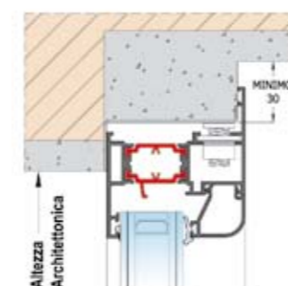
4. Sezione verticale - Nodo superiore fisso
