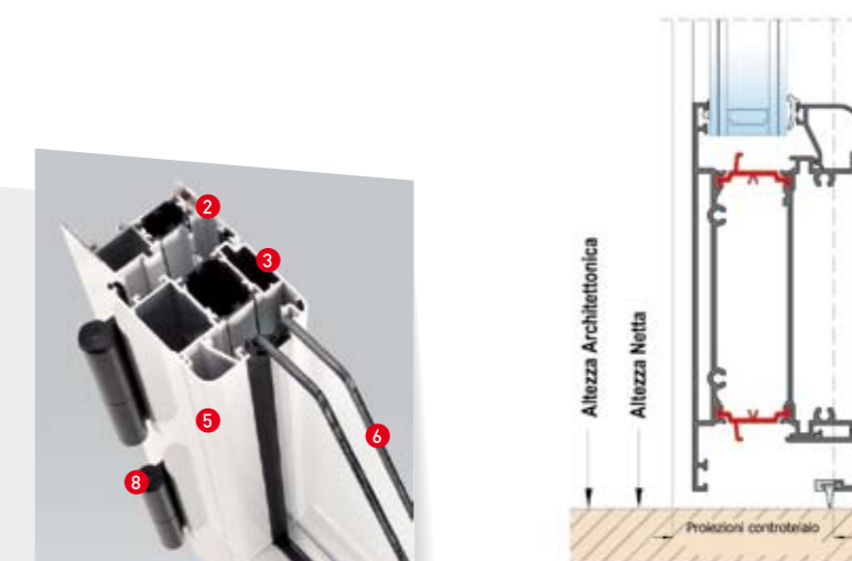
7. Sezione verticale - Nodo inferiore
